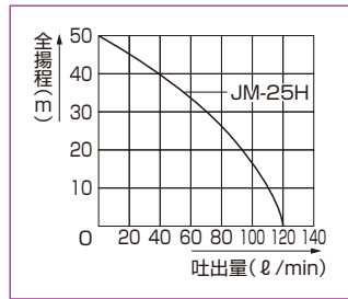
■ 性能曲線
