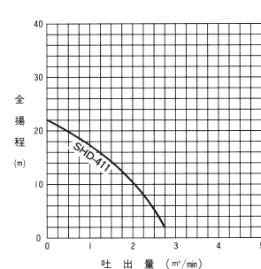
SHD型
