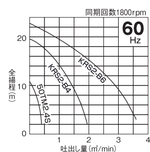
KRS型
