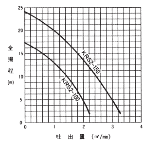
KRS型
