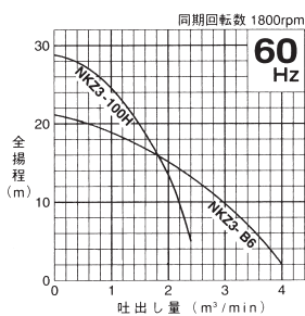
NKZ型
