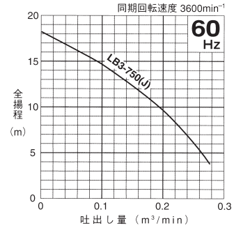
LB3-750(高揚程)
