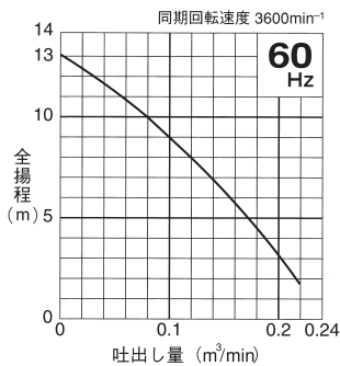
HSD2-55(100V)
