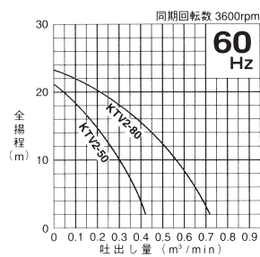
KTV型
