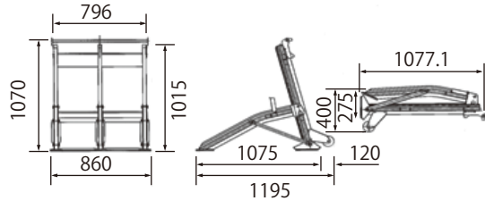
■寸法図
