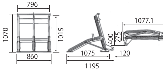
■寸法図
