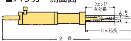
■パッカー側面図
