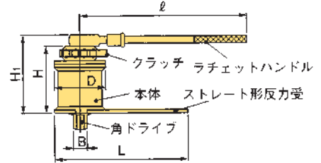
■寸法図 (8-300P)
