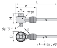
■寸法図 (6-150N)
