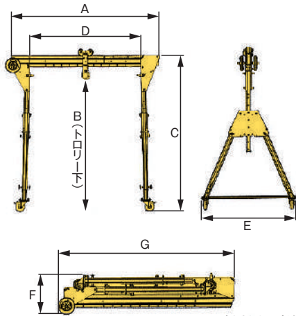
PGR010S-3000、フレーム折りたたみ寸法
