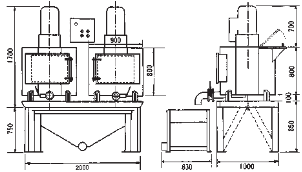
■寸法図（図はNL-400WYです）
