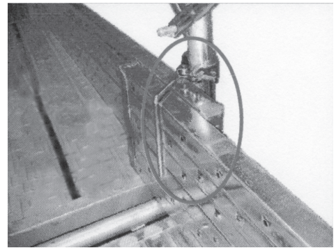
幅木留めクランプ使用例
