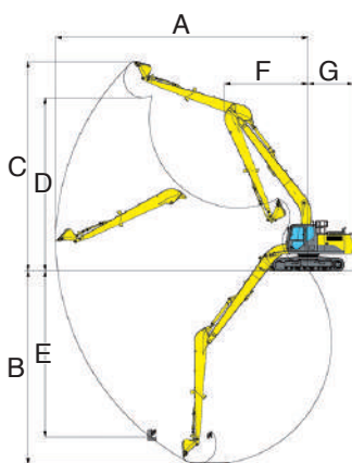
■作業範囲図
